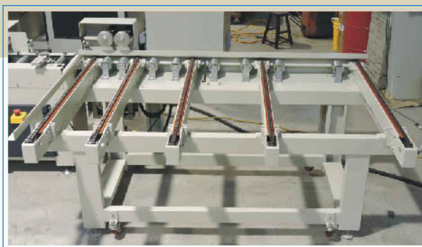
Feeder 進料台
