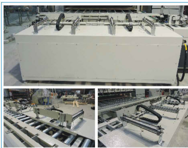
Pusher 推料台
